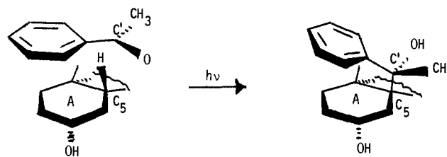
Scheme VI
